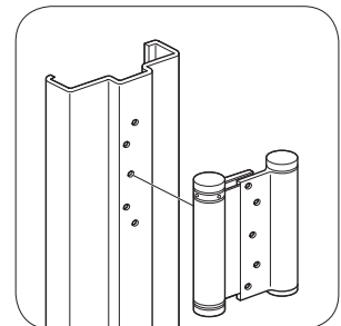
bommer scharnier t.b.v. doordraaideuren
