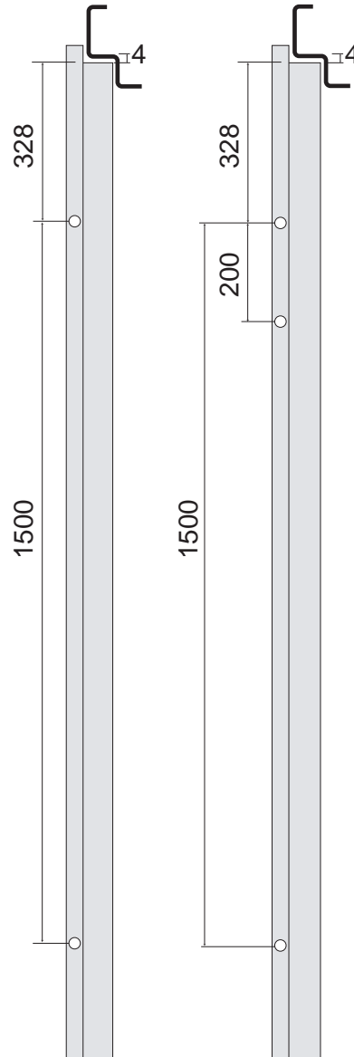
2 paumellen
