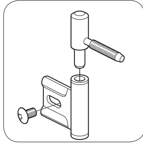
Plus paumelle voor MonoPlus® montagekozijnen, in opdek-uitvoering, verzinkt
